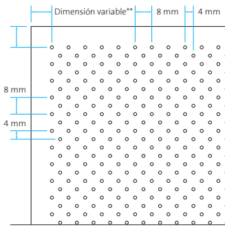
Perforación \varnothing 1,5 mm Área perforada ~ 5,5%
