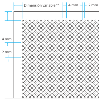
Perforación \varnothing 1,5 mm Área perforada ~ 22%
