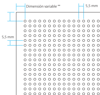
Perforación \varnothing 2,5 mm Área perforada ~ 16%
