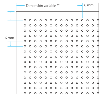
Perforación \varnothing 2 mm Área perforada ~ 9%
