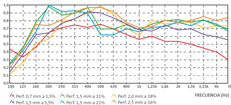
COEFICIENTE DE ABSORCIÓN \alpha_s
