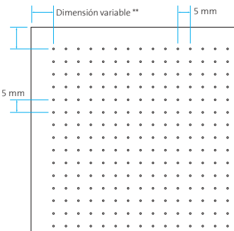
Perforación ultra-micro \varnothing 0,7 mm Área perforada ~ 1,5%
