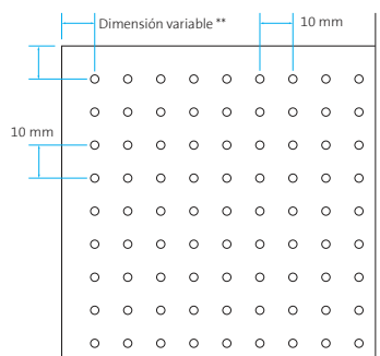
Perforación \varnothing 2,5 mm Área perforada ~ 5%
